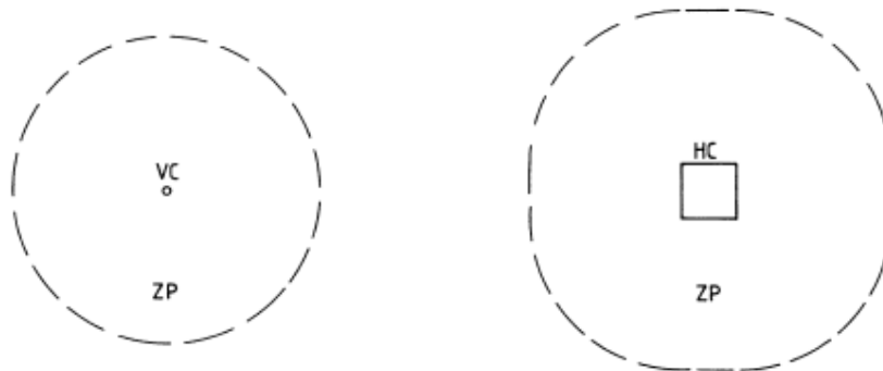
Mặt bằng vùng bảo vệ tại cốt nền
