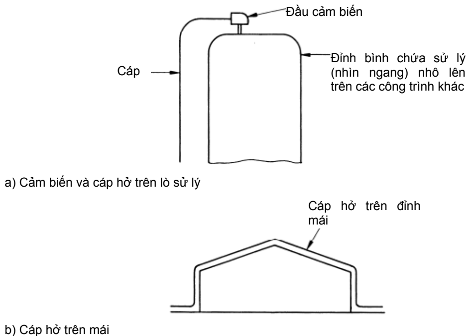
Hình C.11 – Lắp trực tiếp lên hệ thống điện trần ngoài nhà
