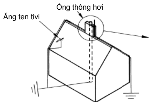
a) Nhà bằng vật liệu không dẫn điện có ăngten tivi trên mái và bộ phận kỹ thuật liên kết với dây xuống
