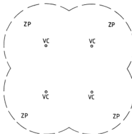
c) Bốn dây dẫn đứng với các góc bảo vệ và vùng bảo vệ kết hợp
