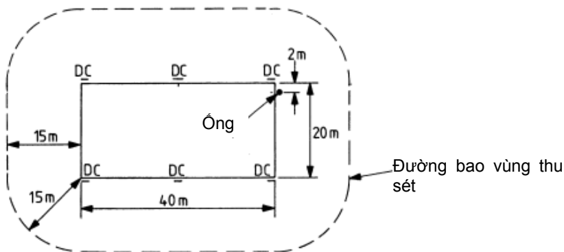
Hình D.1 - Mặt bằng vùng thu sét
