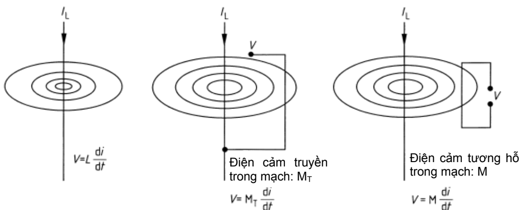
Hình C.17- Điện cảm
