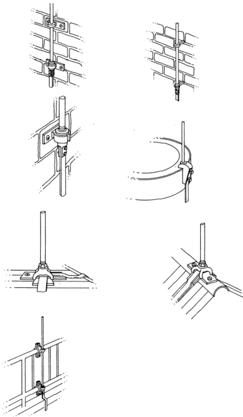
Hình 8. Các kiểu kim thu sét điển hình
