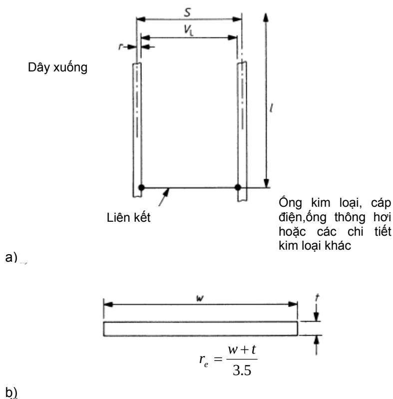
Hình 26. Điện cảm truyền trong mạch đơn giản
