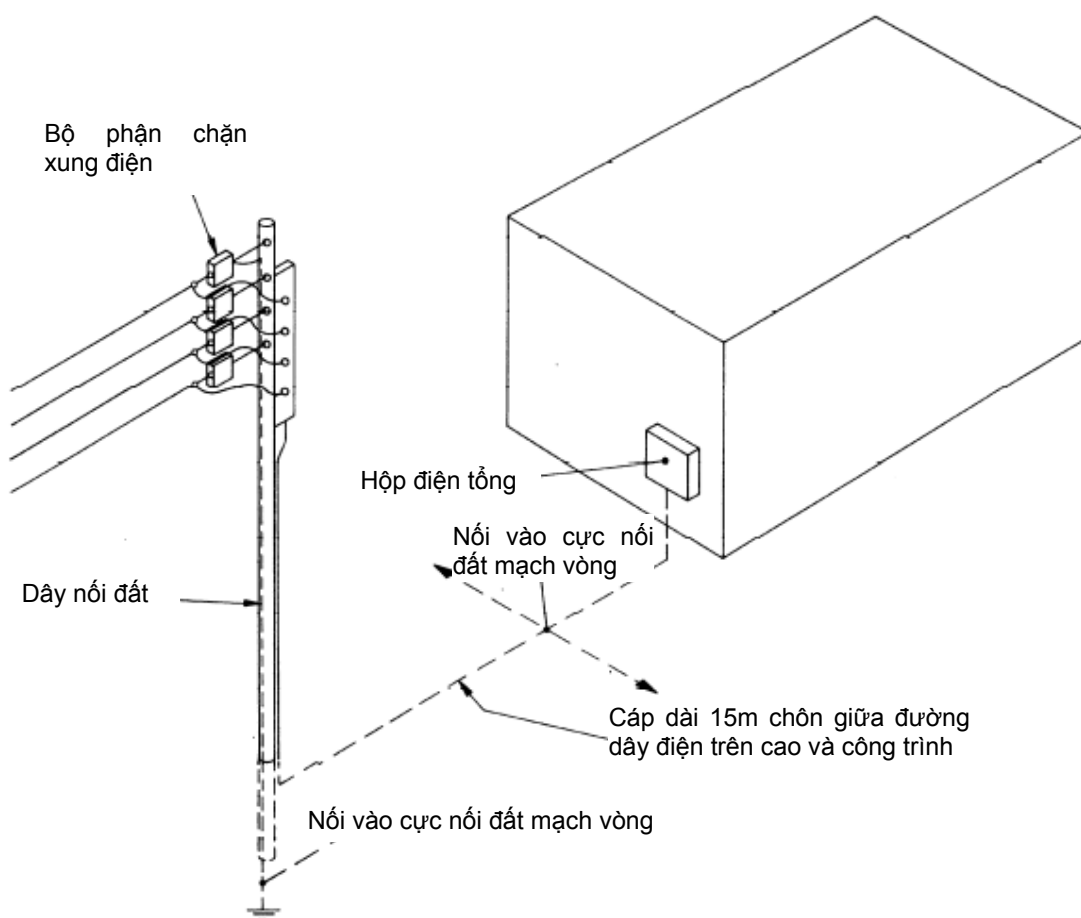
Hình 32. Bảo vệ đặc biệt chống quá dòng do sét gây ra trong nguồn điện cấp vào nhà có chứa chất nổ hoặc chất rất dễ cháy
